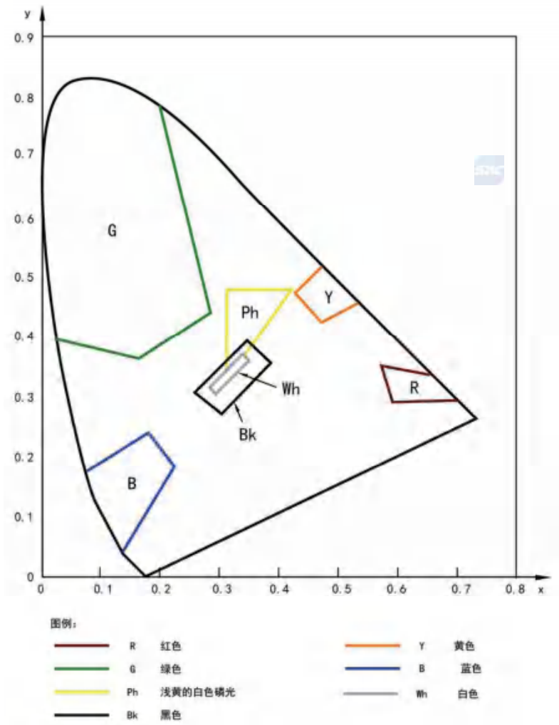
图 A.1 外部照明下的普通材料、磷光材料和未通电的内部照明安全标志的物体色—— 红、黄、绿、蓝、磷光黄白对比、白和黑色的色度边界
